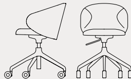
CB2126 56,5x59 H83(73) HS56,5(46,5) HB74,5(64,5) cm
